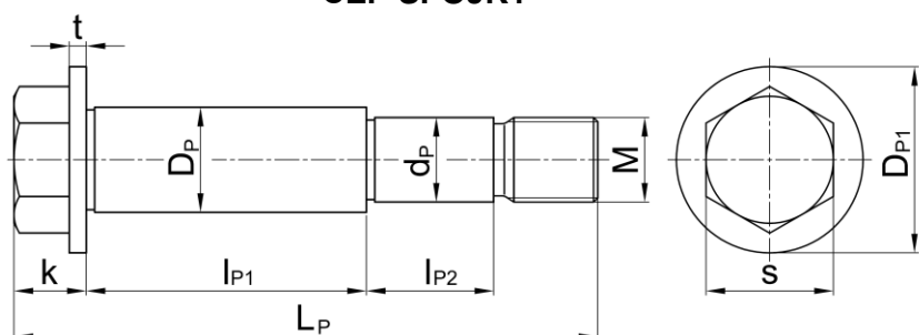
ČEP SPOJKY
