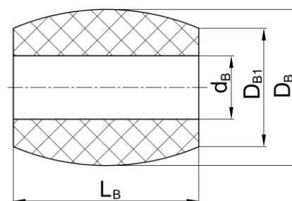
PRYŽOVÉ POUZDRO
