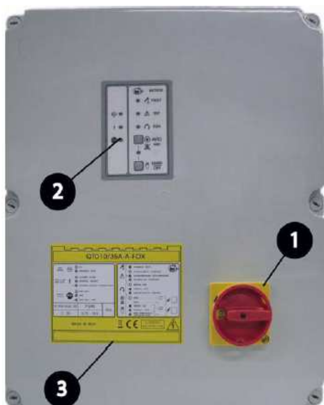
Příklad zařízení QTD10/35A-A-FOX:
