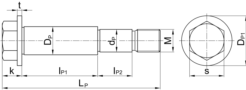
ČEP SPOJKY
